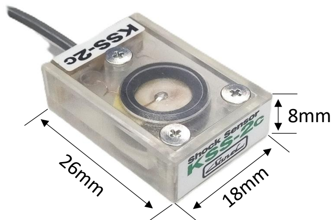
感知部 KSS-2c 表面（前）
