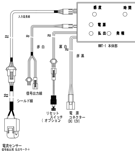
本器の部品接続略図
